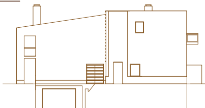
ALÇADO POENTE ALÇADO POENTE ALÇADO POENTE
